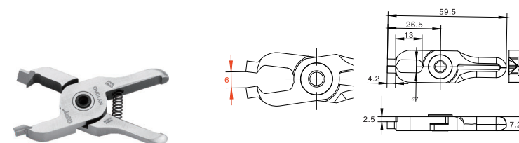
平嘴鉗 Lift blade
