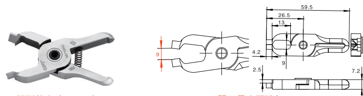
平嘴鉗 Lift blade
