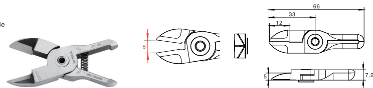
加長平嘴鉗 Straight long blade
